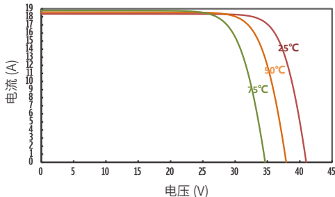
JT600SHk 不同温度下的IV曲线
